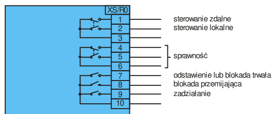
Rys. 35. Przykładowy schemat sygnalizacji w zasilaczu
