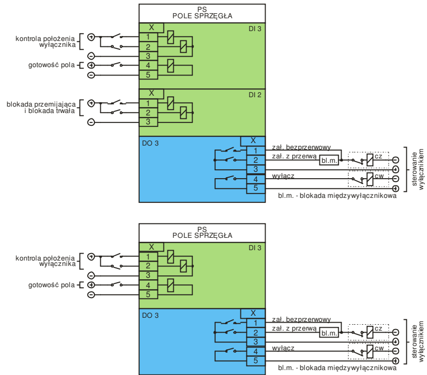
Rys. 37. Przykładowe schematy podłączenia pola sprzęgła
